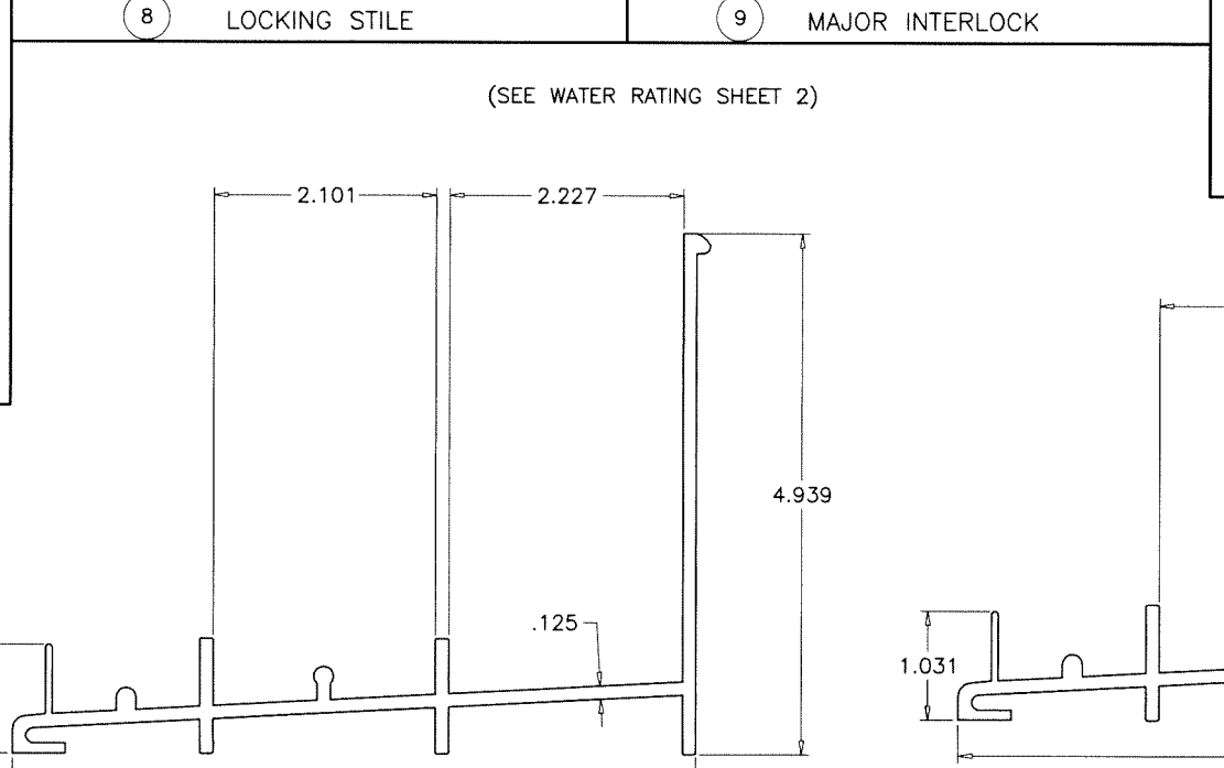
2 2A 2C FRAME SILL
